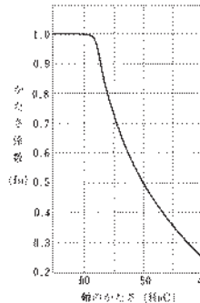
図10：硬さ係数 f_H
