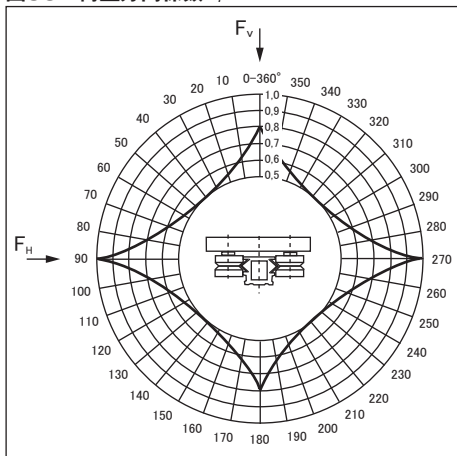
図53：荷重方向係数 f_i
