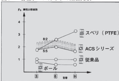
図57：各種クロスガイドの剛性比較
