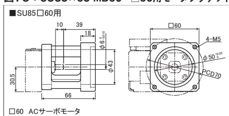
図79：SU85×65-MB60 □60用モータブラケット
