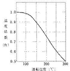
図11：温度係数 f_t
