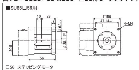
図78：SU85×65-MB56 □56用モータブラケット
