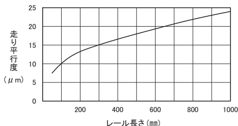
図42：走り平行度
