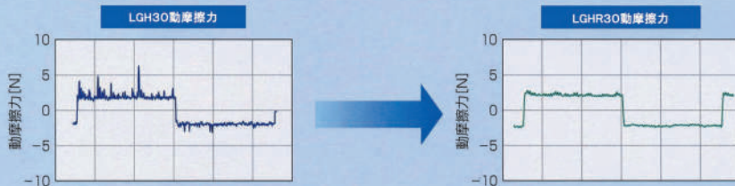
図39：LGHR30とLGSR30の動摩擦力の比較
