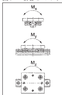
図52：許容モーメント
