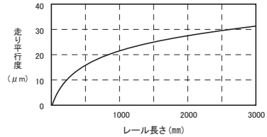
図80：走り平行度
