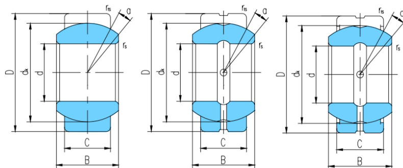
GEG..E
