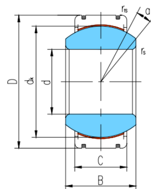
GEG...XT 2RS
