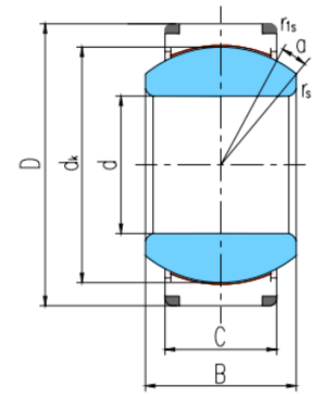
GEH...XT 2RS
