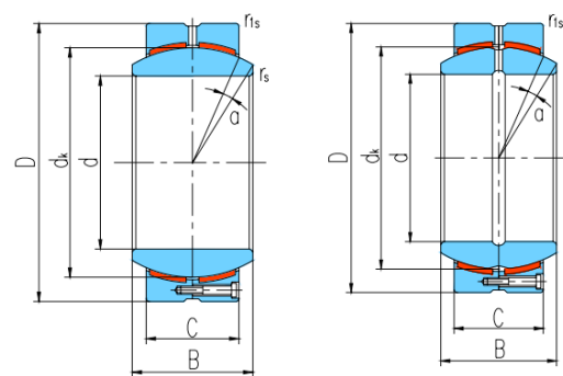
GEH..HC
