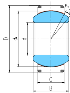
GEH...XT
