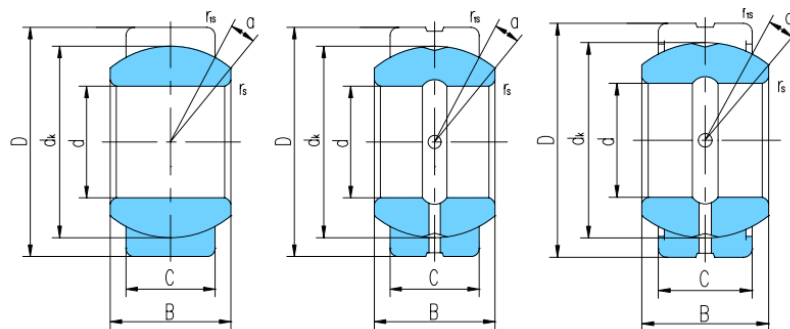
GE..E
